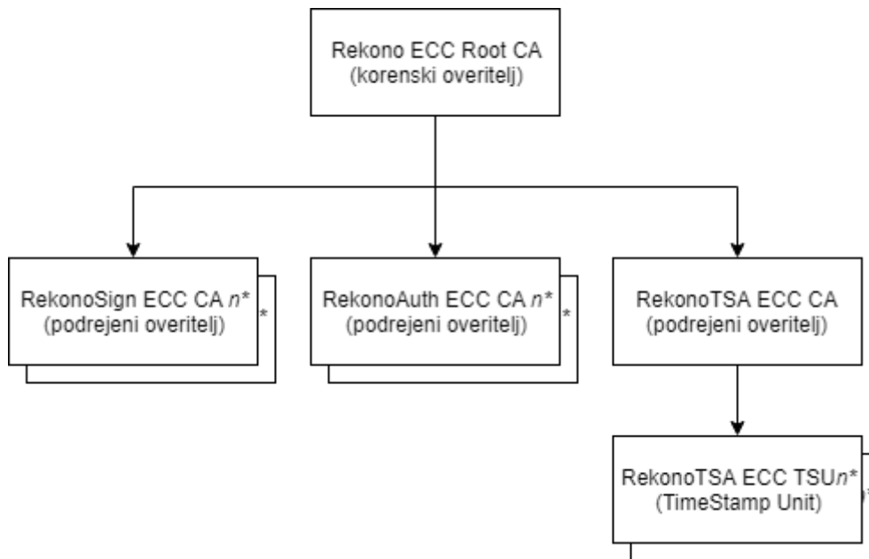
Slika 3 PKI hierarhija overiteljev Rekono TSP v verigi zaupanja s ključi ECC
