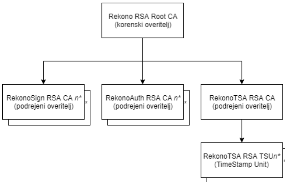
Slika 2 PKI hierarhija overiteljev Rekono TSP v verigi zaupanja s ključi RSA
